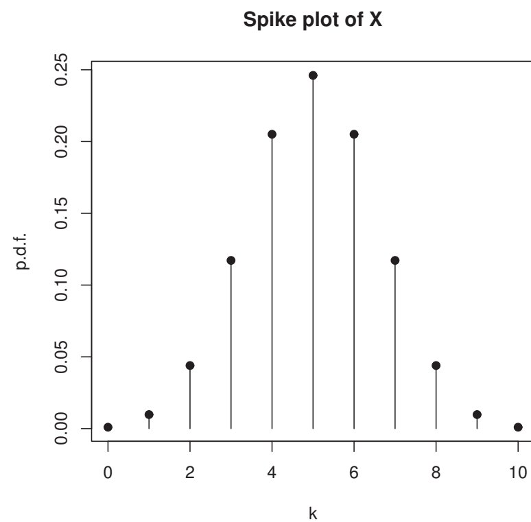
Figure 3: 2 項分布の確率関数のグラフ ( n = 10, p = 1/2 )
