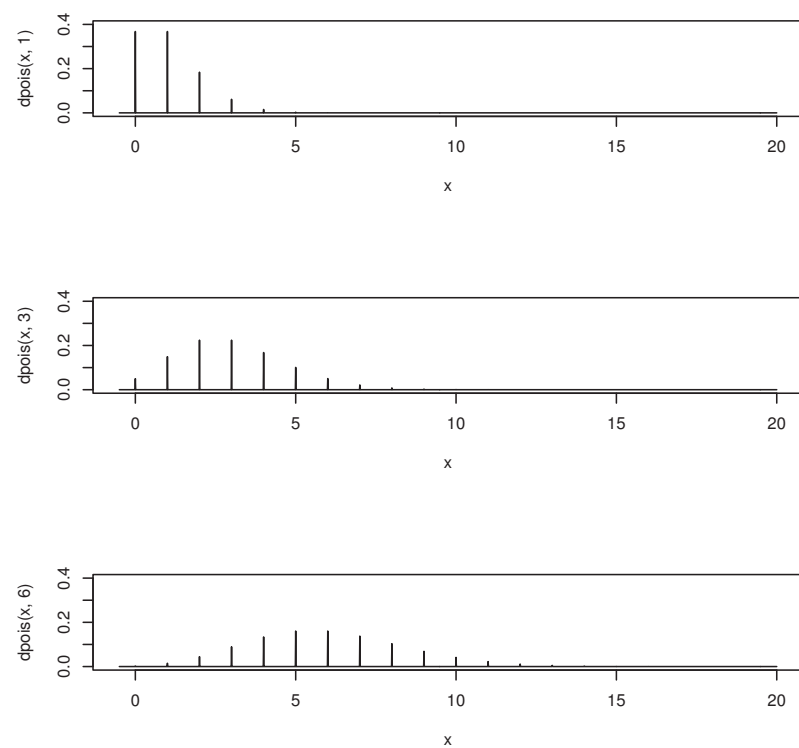
Figure 4: ポアソン分布の確率関数のグラフ ( \lambda = 1, 3, 6 )
