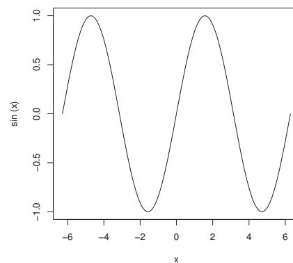
Figure 6: 正弦関数のグラフ
