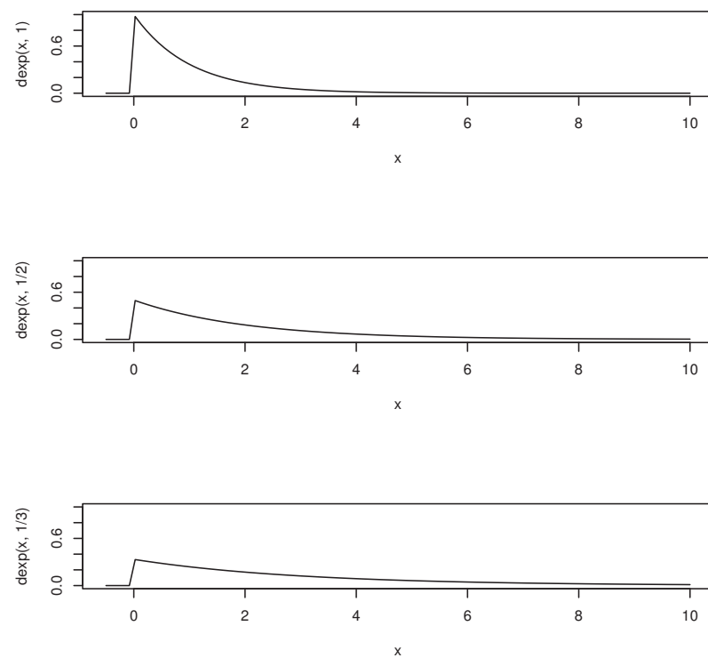
Figure 10: 指数の確率密度関数のグラフ ( \lambda = 1, 1/2, 1/3 )
