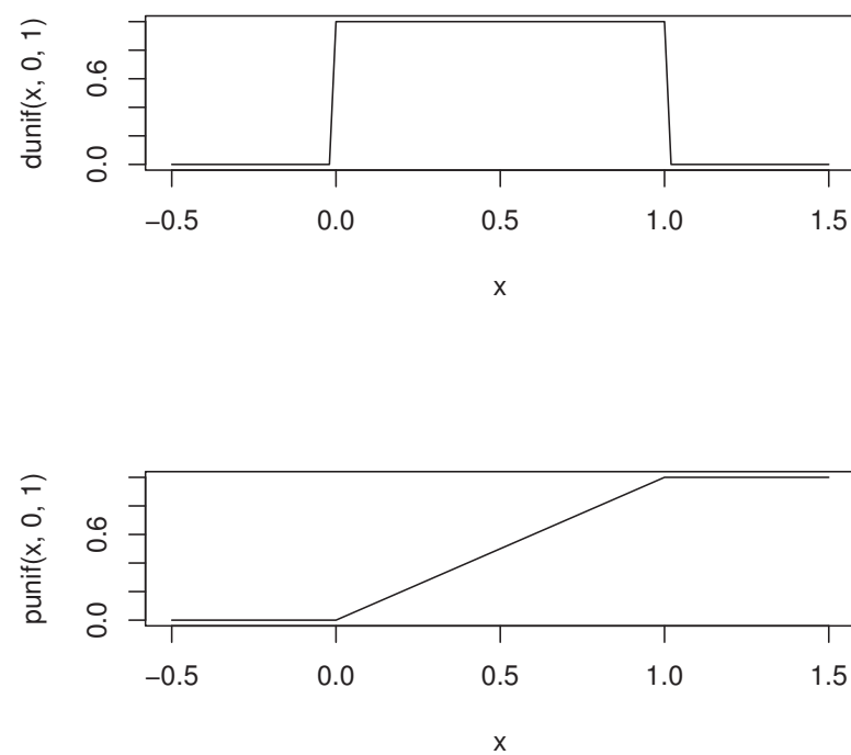
Figure 9: 一様分布の確率密度関数と累積分布関数のグラフ
