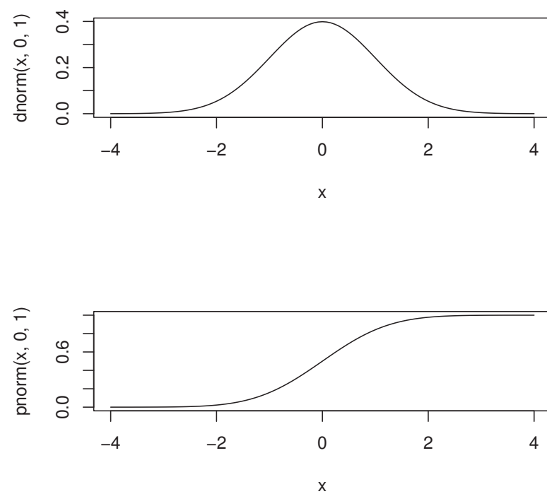
Figure 7: 標準正規分布の確率密度関数と累積分布関数のグラフ
