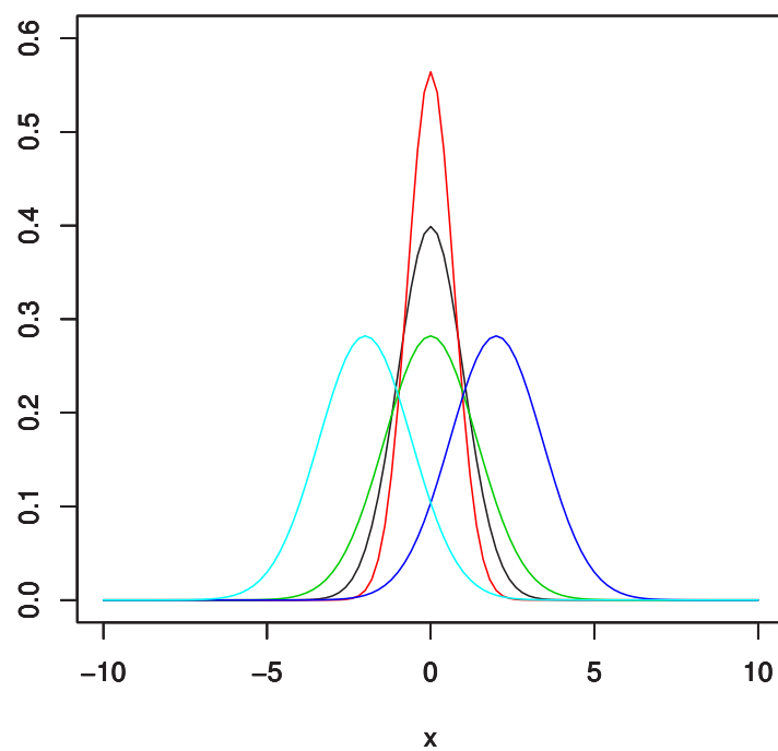
Figure 8: N(0, 1) , N(0, 2) , N(0, 1/2) , N(2, 2) , N(-2, 2) の確率密度関数のグラフ
