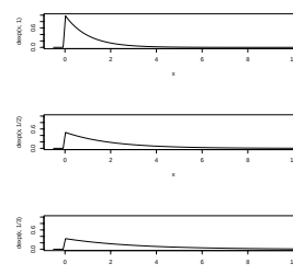
Figure 8: 指数の確率密度関数のグラフ ( \lambda = 1, 1/2, 1/3 )
