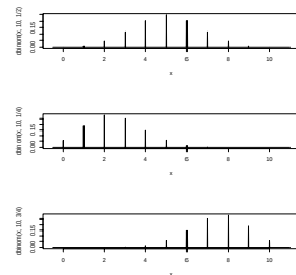
Figure 2: 2 項分布の確率関数のグラフ ( n = 10, p = 1/2, 1/4, 3/4 )
