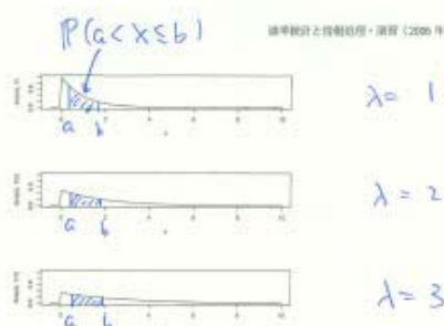
Figure 8: 指数の確率密度関数のグラフ ( \lambda = 1, 2, 3 )
