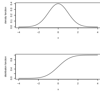
Figure 1: 連続型確率変数の確率密度関数 (上) と分布関数 (下)
