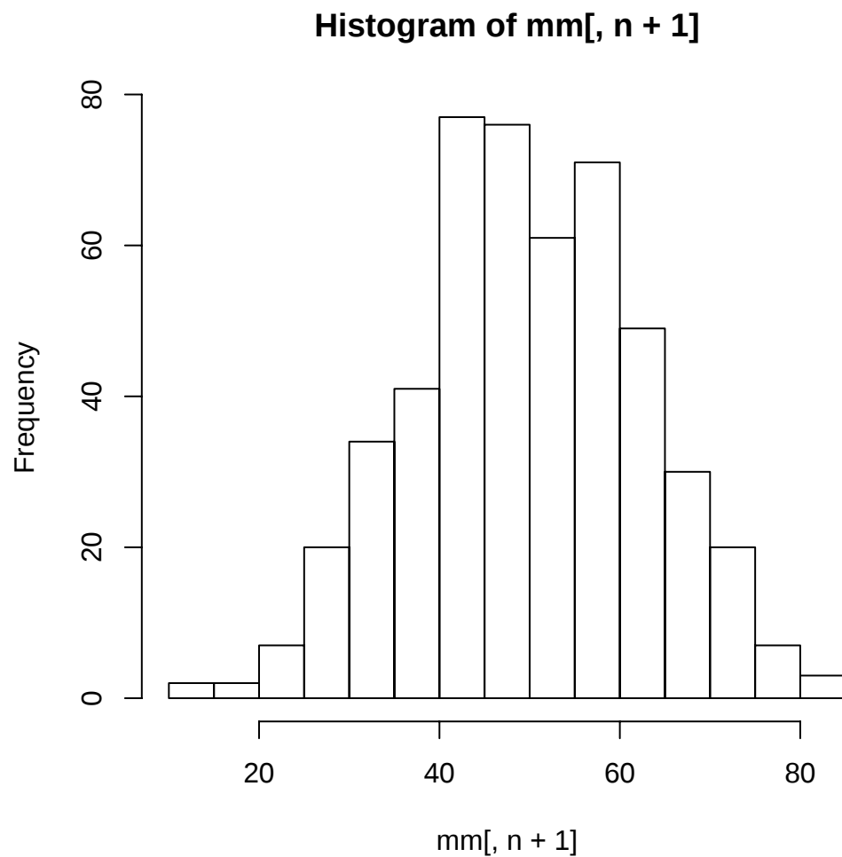
Figure 1: n = 5 のときの標本平均のヒストグラム ( 平均 = 51.0424, 標準偏差 6 = 12.30351 )
